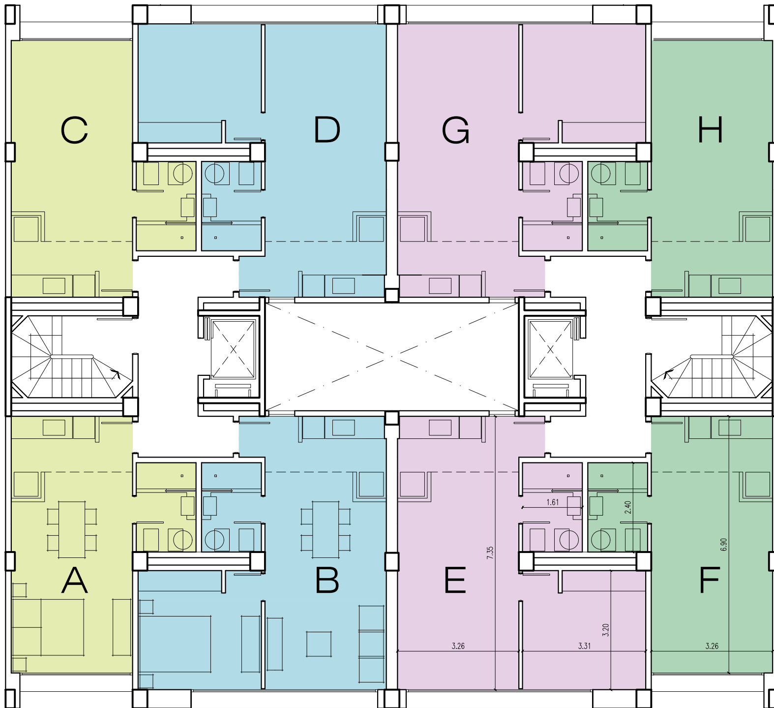
PLANTA 2° PISO
