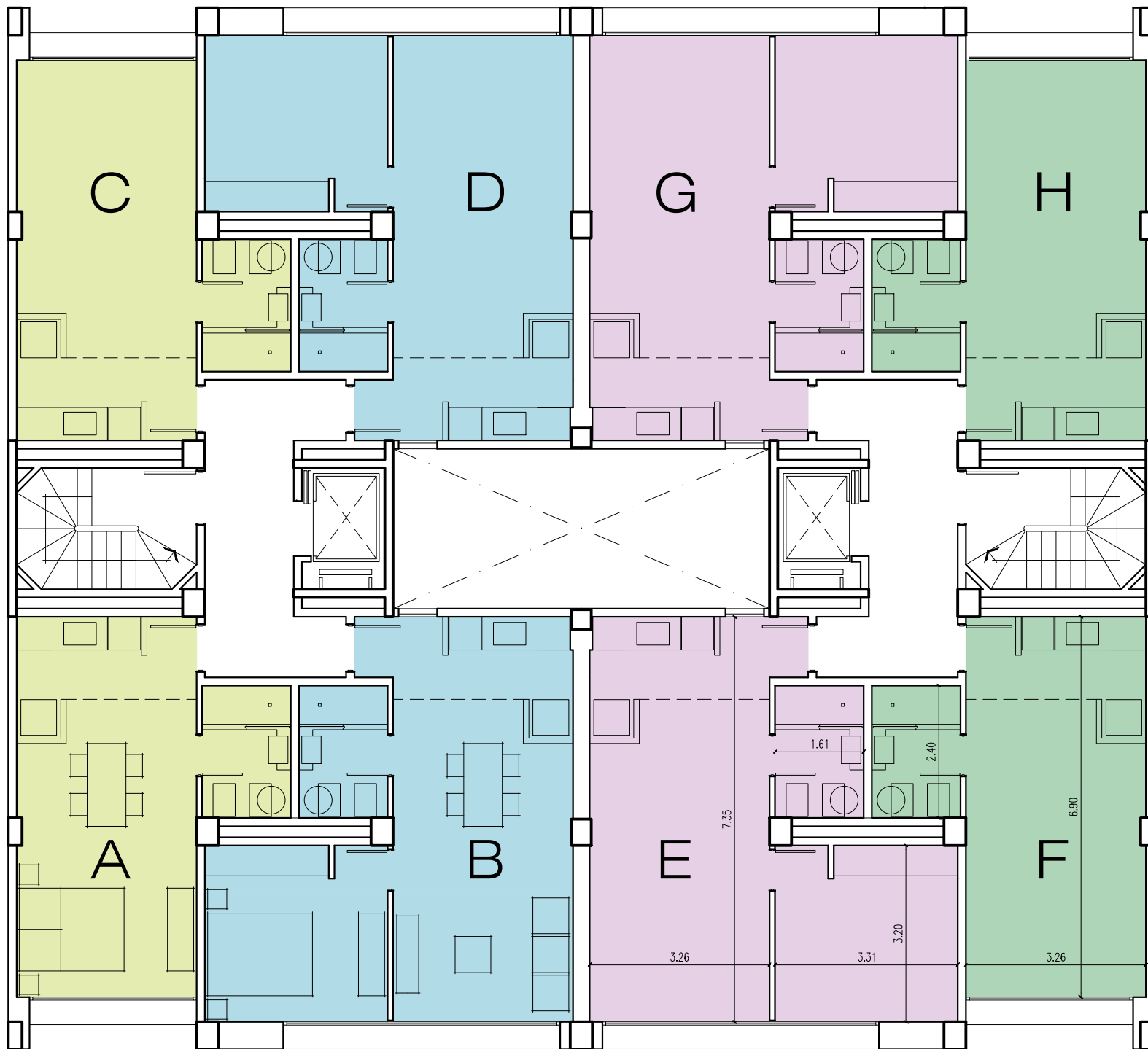
PLANTA 3° PISO
