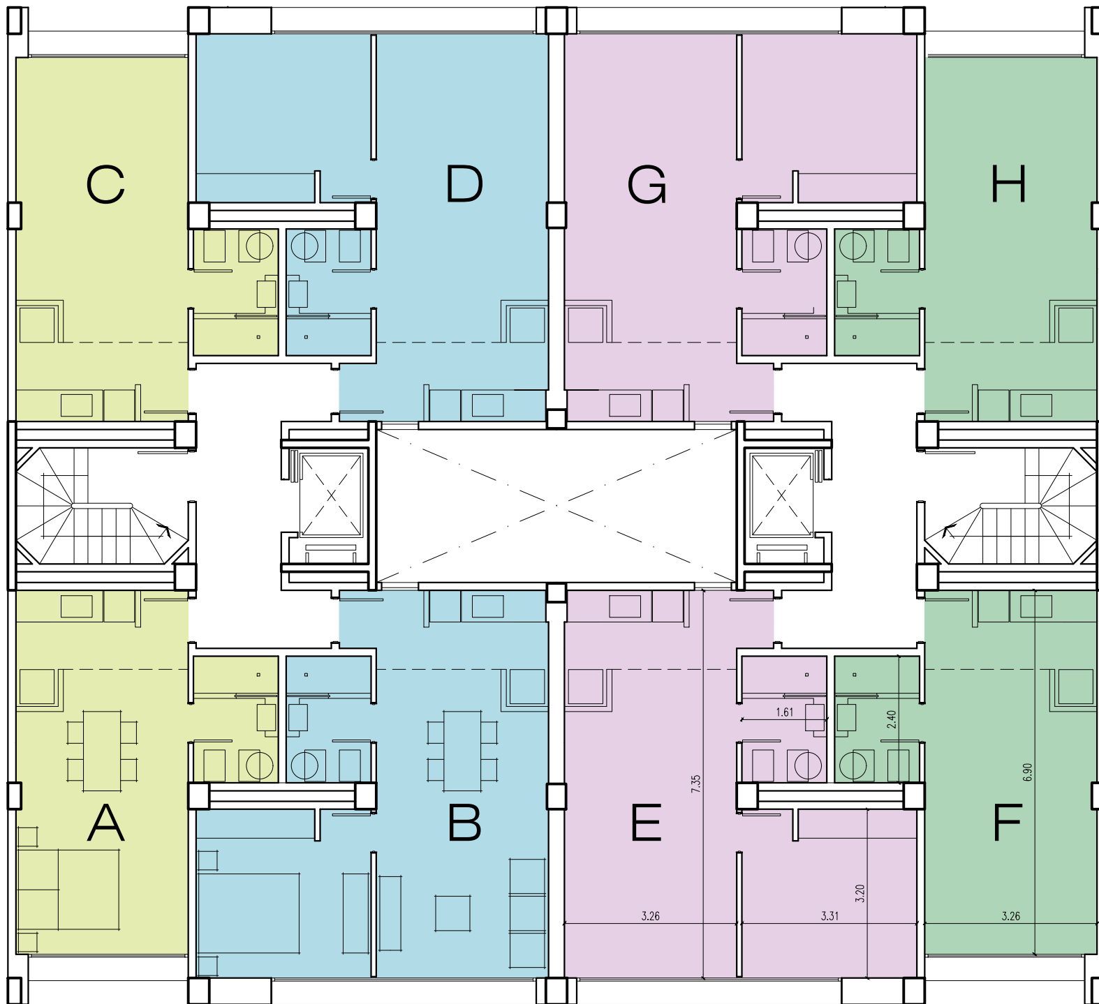
PLANTA 6° PISO
