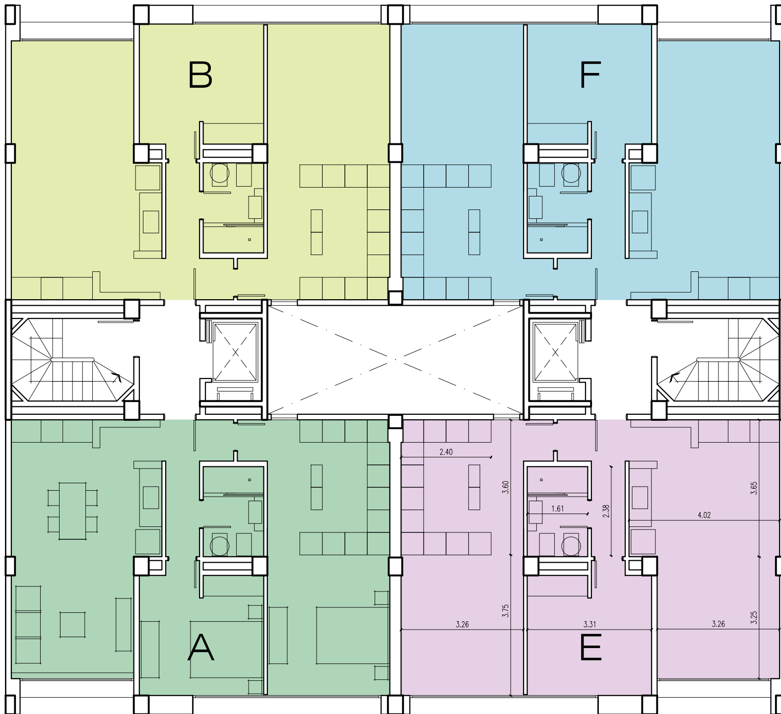
PLANTA 7° PISO
